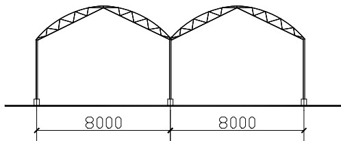
变截面桁架
