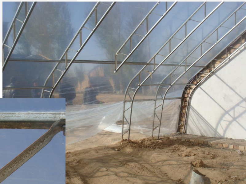
槽钢弦杆-型钢腹杆
